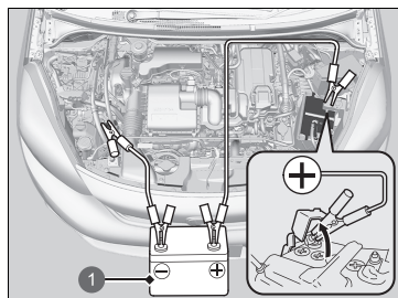
1 Batterie d'appoint
